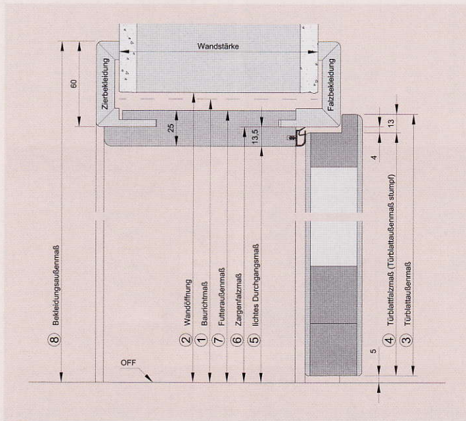
Vertikalschnitt vertical cut
