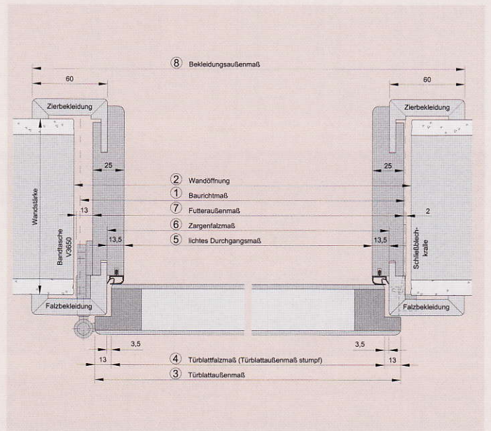
Horizontalschnitt einflügelig horizontal cut single leaf
